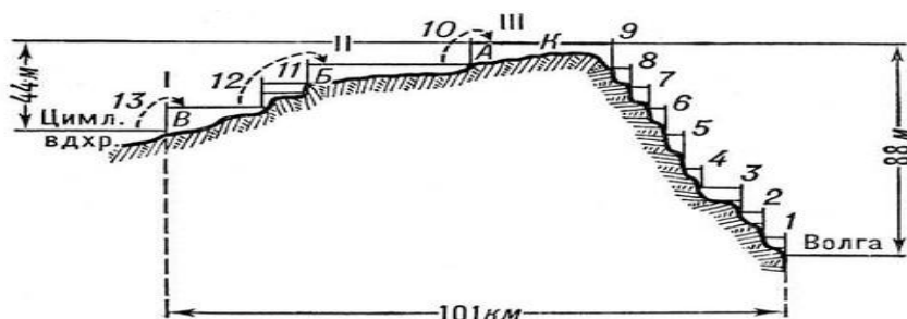
Рисунок 1 Схема канала в разрезе
